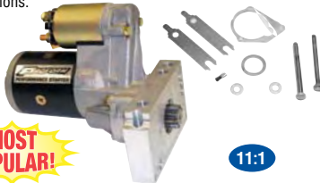
66256.....12V 1.4 KW motor
